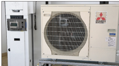
Eine moderne Wärmepumpe mit Brennwertgerät.
